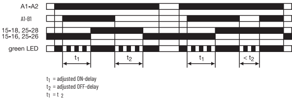
(D) Impulse-ON
